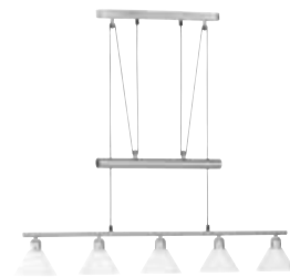
Pendelleuchte · Pendant ↔ 102 x 14 cm, ↓ 80 - 180 cm excl. 5 x E14, max. 40 W
