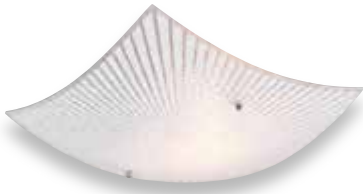
Deckenleuchte · Ceiling lamp ↔ 30 x 30 cm, ↓ 9 cm excl. 1 x E27, max. 40 W
